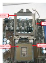
1155 針插槽圖
