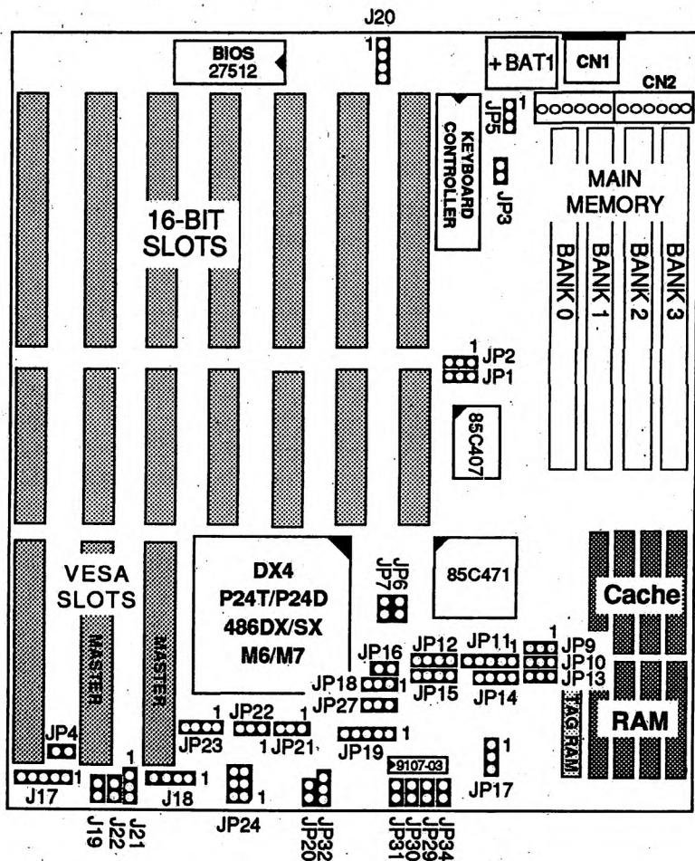
Abbildung 1-1. Mainboard Layout
