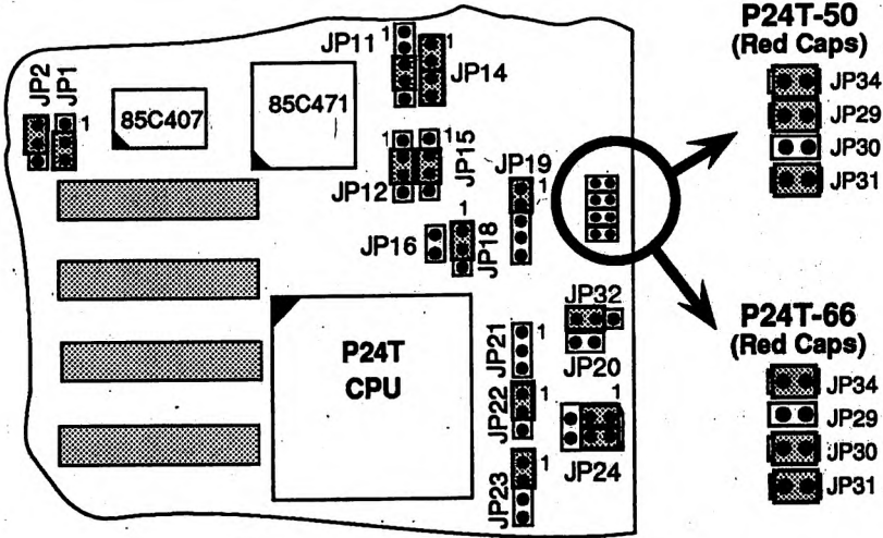
Abbildung 2-6. Jumper Stellung P24T-50/66
