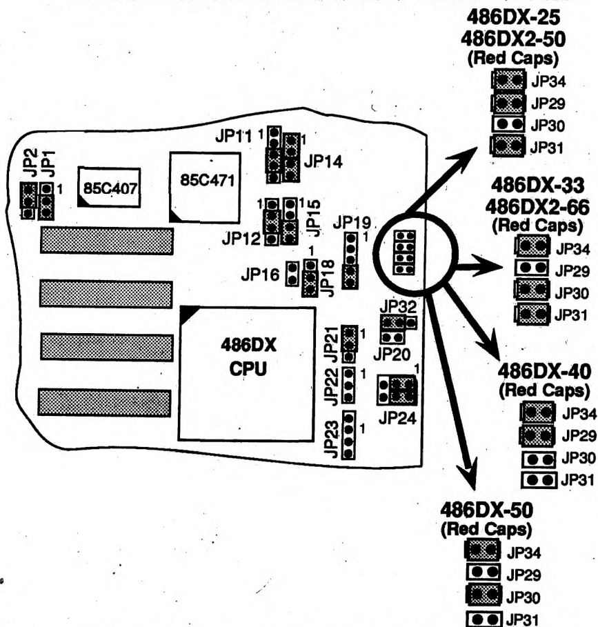
Abbildung 2-3. Jumper Stellung für 486DX-25/33/40/50, 486DX2-50/66
