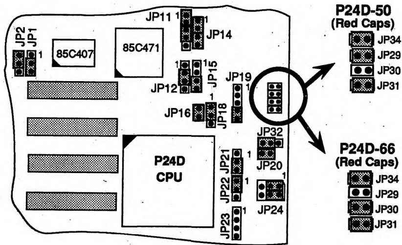
Abbildung 2-7. Jumper Stellung P24D-50/66
