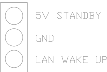
Fig. 7 LAN Wake Up Connector
