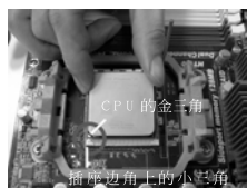
步骤 2 / 步骤 3： 将 CPU 的金三角对准插座 边角上的小三角
