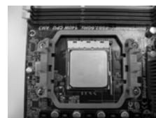
PASO 4: Apriete Hacia Abajo y Bloquee La Palanca del Zócalo
