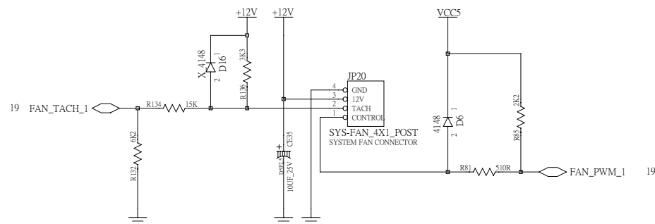
Chassis FAN for CPU
