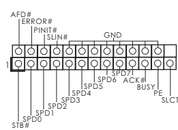
打印机端口接针 (25 针 LPT1) (见第 2 页第 21 项)
