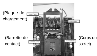
Vue d'ensemble du socket 1156 broches
