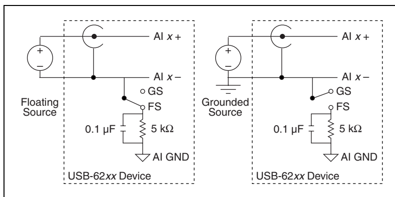
Figure A-7. Analog Input Circuitry
