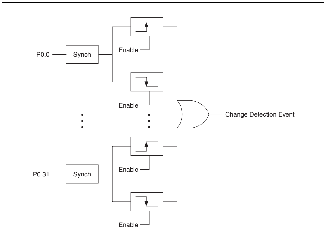
Figure 6-3. DI Change Detection
