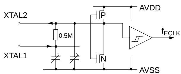
Fig. 3-8: Crystal Oscillator
