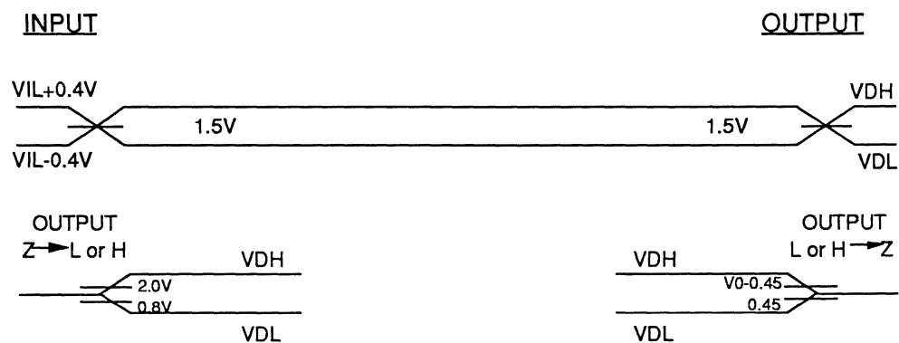
FIG. 15 A.C. TESTING INPUT, OUTPUT
