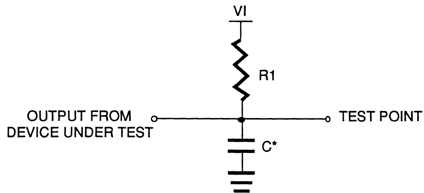
FIG. 14 A.C. TEST CIRCUITS
