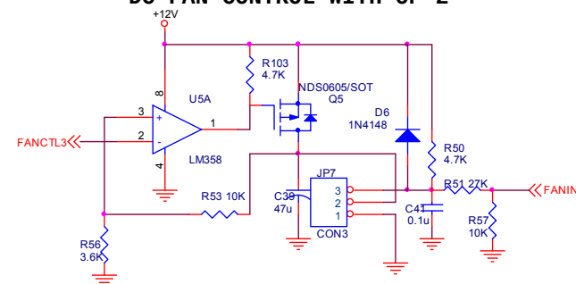
DC FAN CONTROL WITH OP 3
