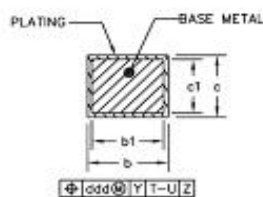
SECTION G-G SCALE: 100/1
