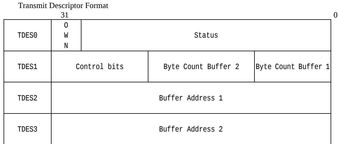
Fig - 5 Transmit Descriptor Format
